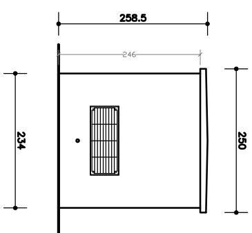
PROSPETTO B
