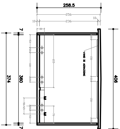
SEZIONE X-X
