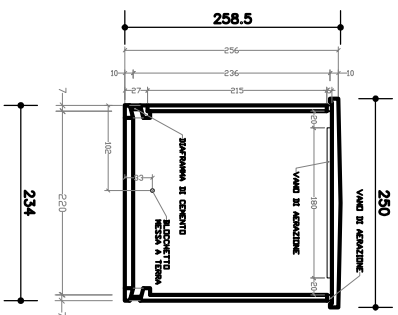
SEZIONE F-F
