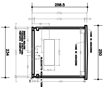
SEZIONE E-E
